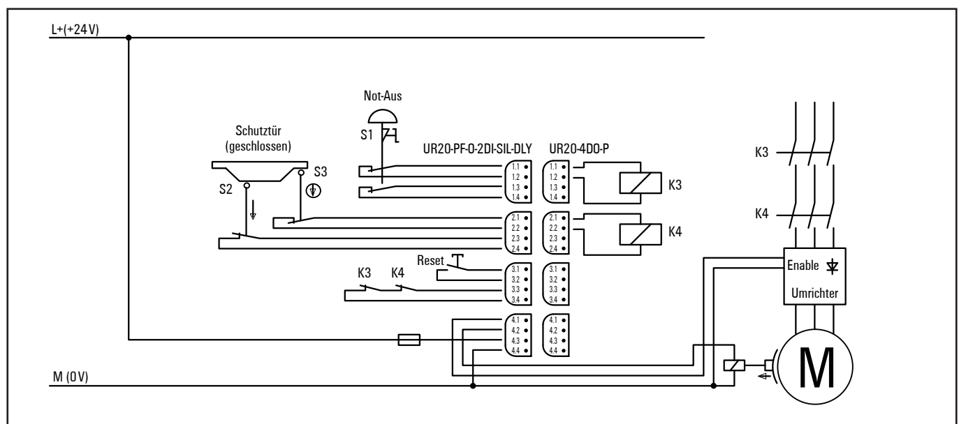
Beispielapplikation zweikanalige Schutztürüberwachung mit automatischem Reset und gesteuertem Stillsetzen und Not-Halt
