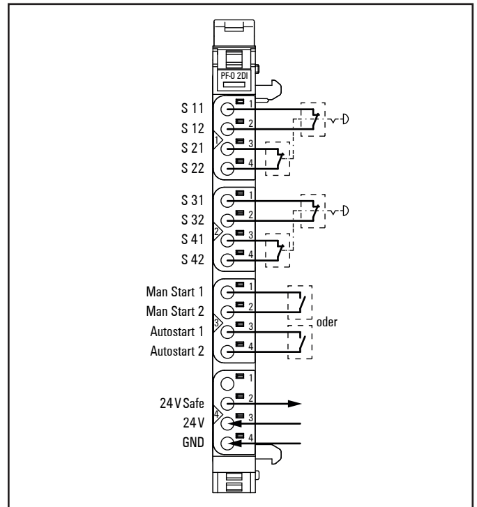
Anschlussbild UR20-PF-O-2DI-SIL
