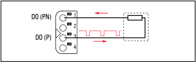
Anschlussbeispiel Interface Typ D – Quelle
