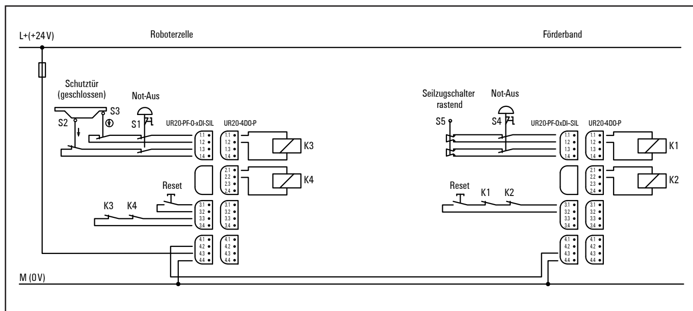
Beispielapplikation Kaskadierung
