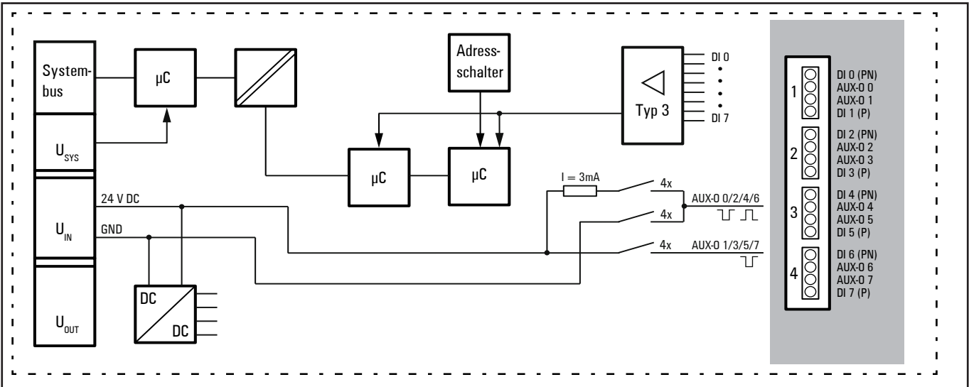
Blockschaltbild UR20-8DI-PN-FSCC
