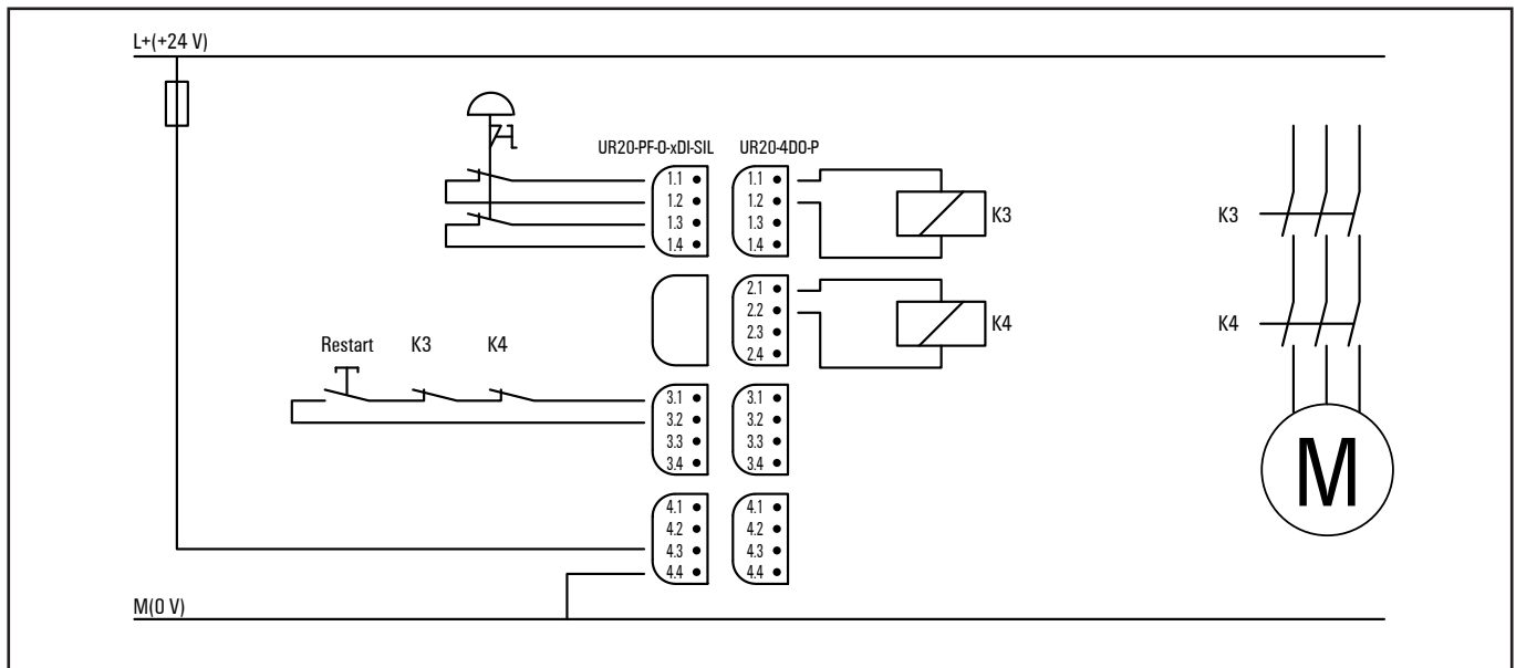
Beispielapplikation 2-kanalige Not-Halt-Überwachung
