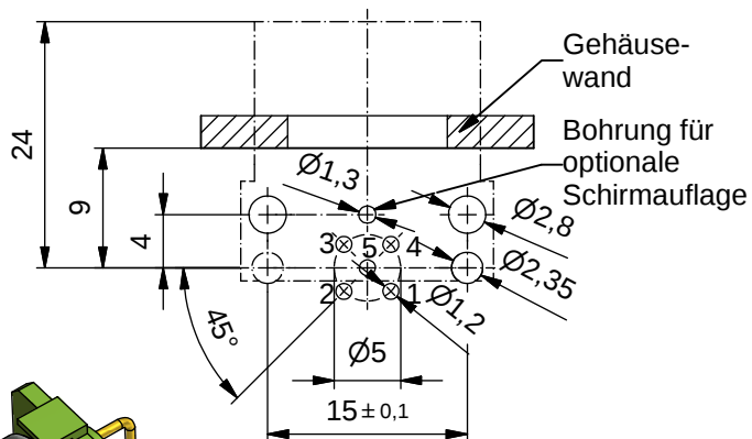
Lochbild Leiterplatte Leiterplatte 1,60mm
