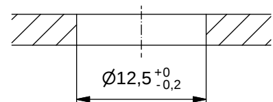
Durchgangsloch
