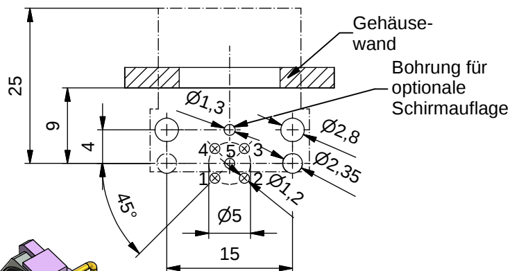
Lochbild Leiterplatte Leiterplatte 1,60mm
