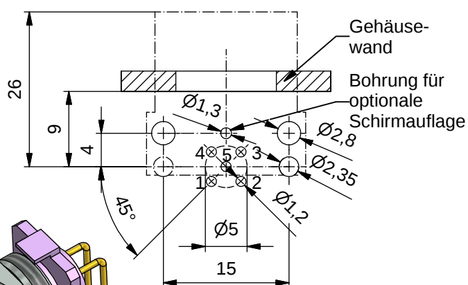
Lochbild Leiterplatte Leiterplatte 1,60mm
