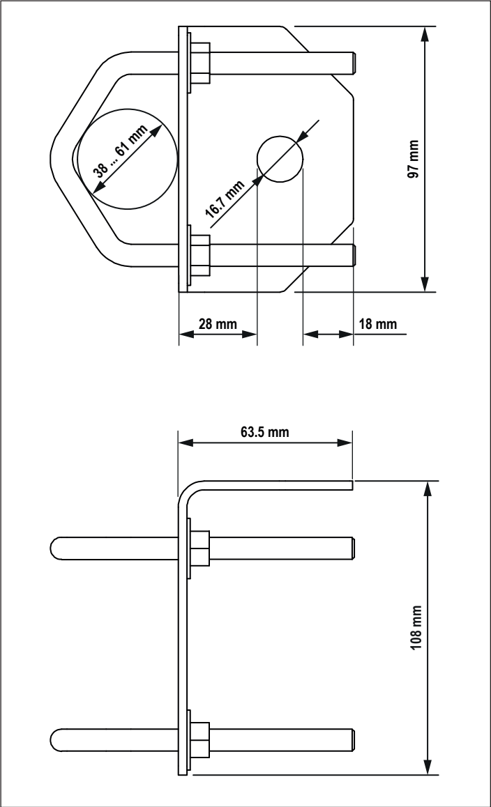
Maße / Dimensions
