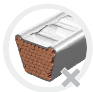
Rissbildung oder Aufplatzen an den Seitenkanten
