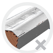
Rissbildung an den Abdrücken des Crimpstempels
