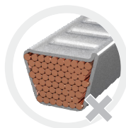
Unsymmetrische Crimpform. Einseitige Gratbildung
