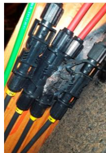
Abbildung 2: Beispiel für Schmorstellen an den Steckverbindern
